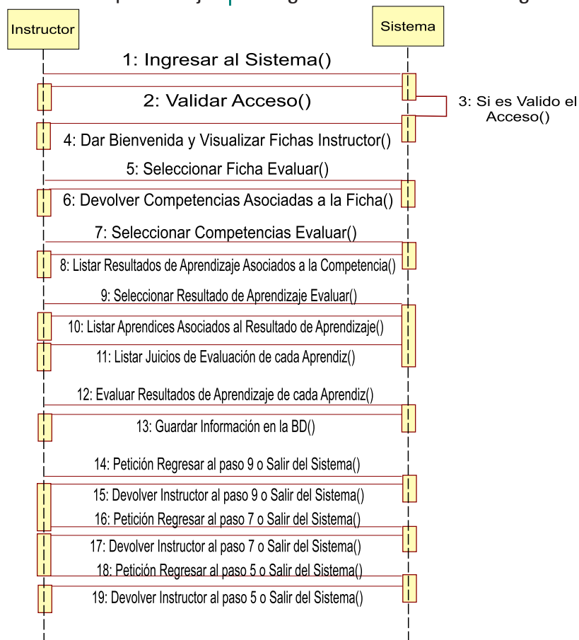
Figura 2. Caso de uso Evaluar, Diagrama de Secuencia Evaluar resultados de aprendizaje
