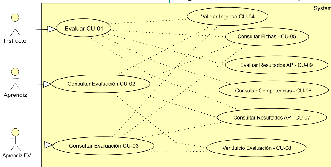
Figura 1. Casos de Uso Sistema GEVA.
