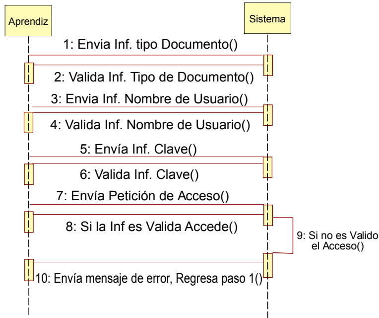
Figura 5. Caso de uso validar ingreso, Diagrama
