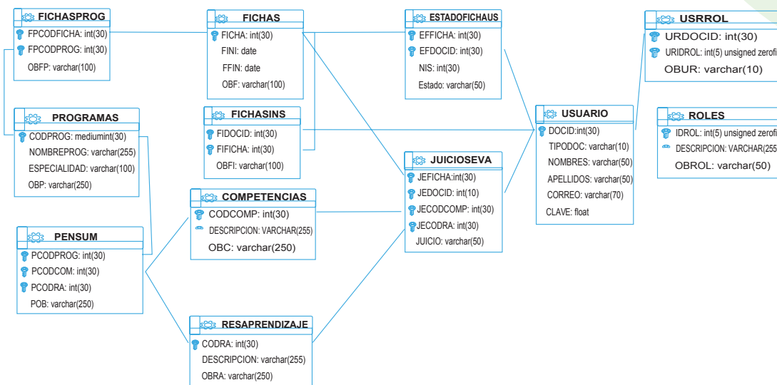
Figura 11. Modelo Relacional de la Base de Datos
