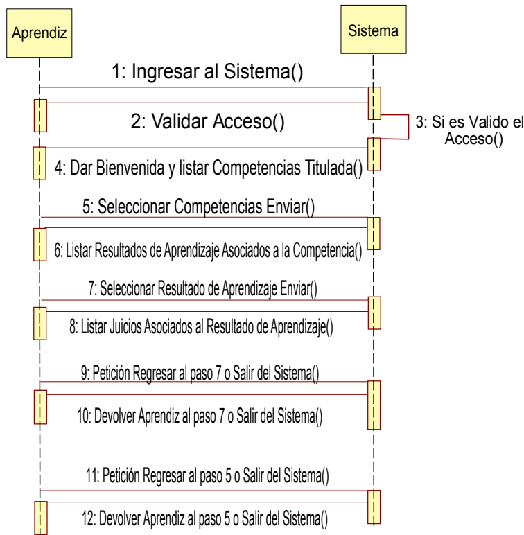
Figura 6. Caso de uso consultar resultados,
