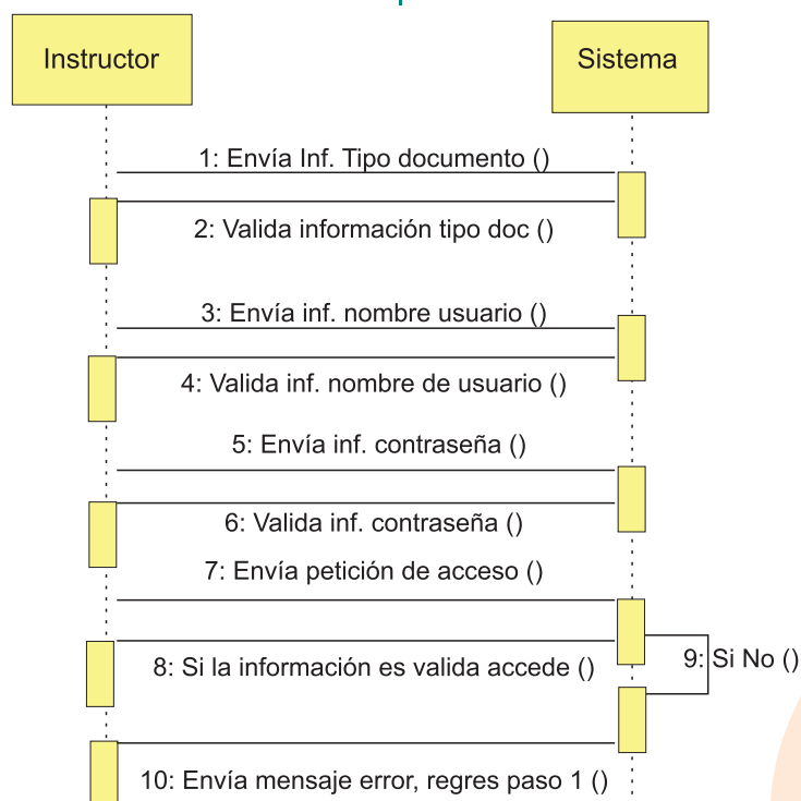
Figura 3. Caso de uso validar ingreso, Diagrama de Secuencia Validar Ingreso del Instructor
