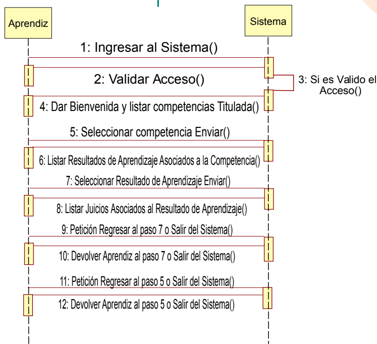
Figura 4. Caso de uso consultar resultados, Diagrama de Secuencia Consultar Juicios Evaluativos
