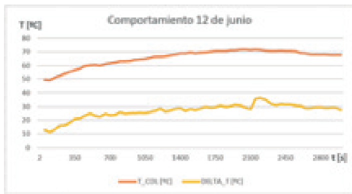
Figura 2. Variación de las temperaturas a lo largo del tiempo: T_COL corresponde a la temperatura promedio en el absorbedor y DELTA_T corresponde a la diferencia de temperatura entre T_COL y la temperatura ambiente.
