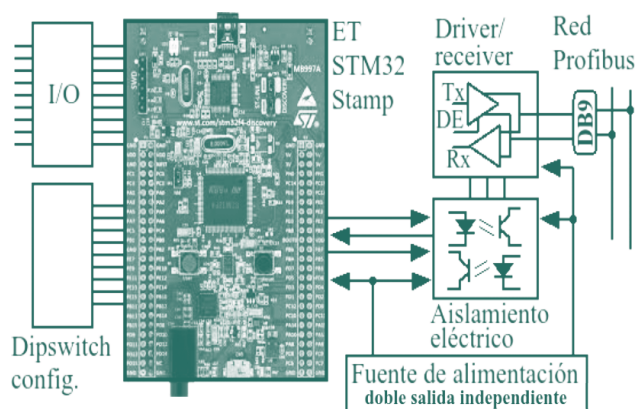
Figura 1. Diagrama de bloques del hardware del esclavo Fuente: Los autores
