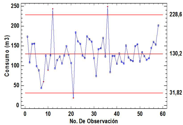
Figura 2. Carta de Control de Individuales para Bloque ABC Fuente: elaboración propia.
