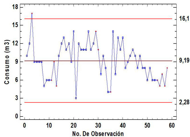
Figura 5. Carta de Control de individuales para Bloque I Fuente: elaboración propia.
