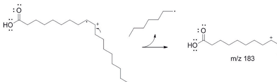
Figura 9. Ruptura en doble enlace Fuente: elaboración propia.
