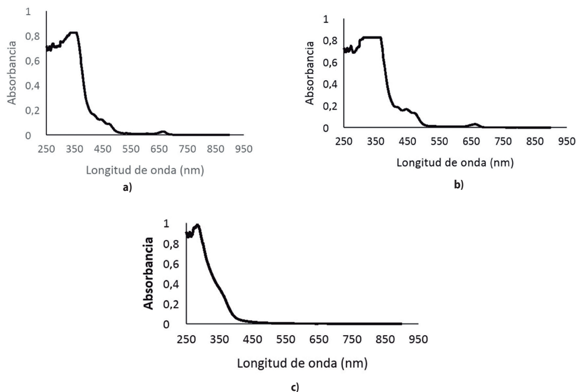
Figura 2. Espectros de absorción de extractos etanólicos obtenidos a diferentes temperaturas de secado de las hojas de P. americana :
