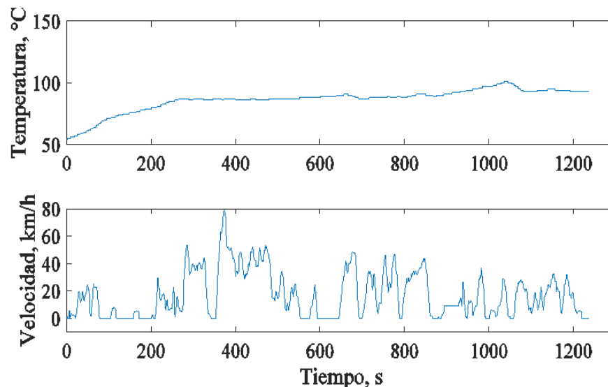
Figura 3. Señal de temperatura del refrigerante del motor durante un recorrido del vehículo
