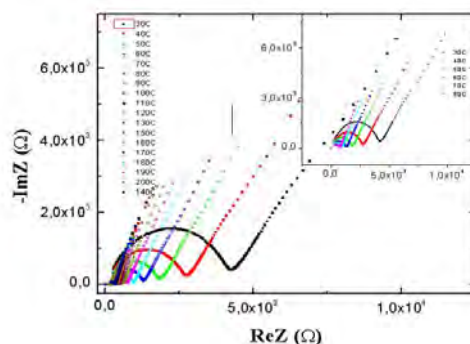
Gráfica 1. Diagrama de Nyquist de la muestra de PVA:CS (80:20) +0.5 H_3PO_2
