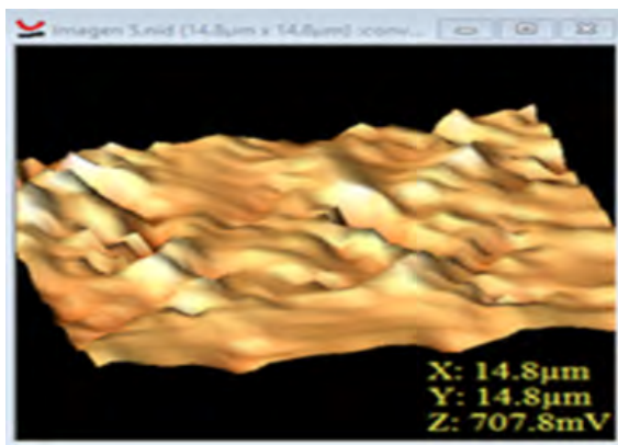
Figura 3. Imagen de AFM del biopolímero obtenido con cáscara de papa modo contacto.
