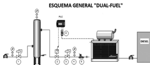
Figura 3. Esquemático dual-fuel usando gas de pozo y Scrubber en un motor diesel.
