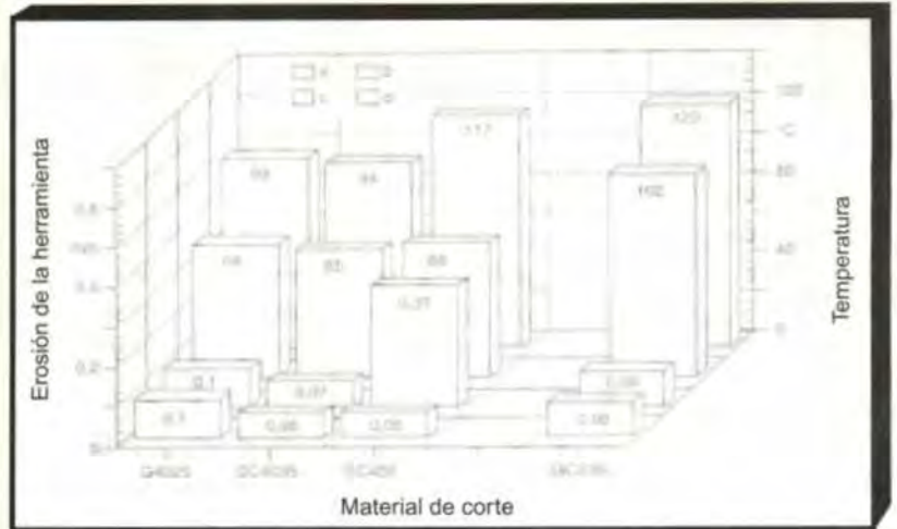
Figura 5. Comparación entre maquinado seco y húmedo al torneado C54, a) desgaste de la herramienta en el torneado húmedo b) en el torneado seco c) temperatura del inserto d) de la pieza
