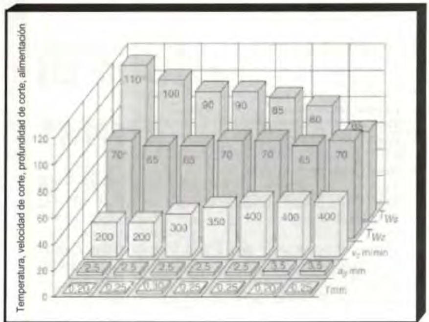
Figura 6. Temperatura de pieza y herramienta en función del porcentaje de desprendimiento de viruta que en el torneado seco (material C45, brillante, 50x80 mm, pieza terminada 20 x 80 mm, volumen removido V 130 cm3, material de corte M25/K20; profundidad de corte y alimentación; Vc velocidad de corte, Tws temperatura de la pieza y Twz temperatura de la herramienta
